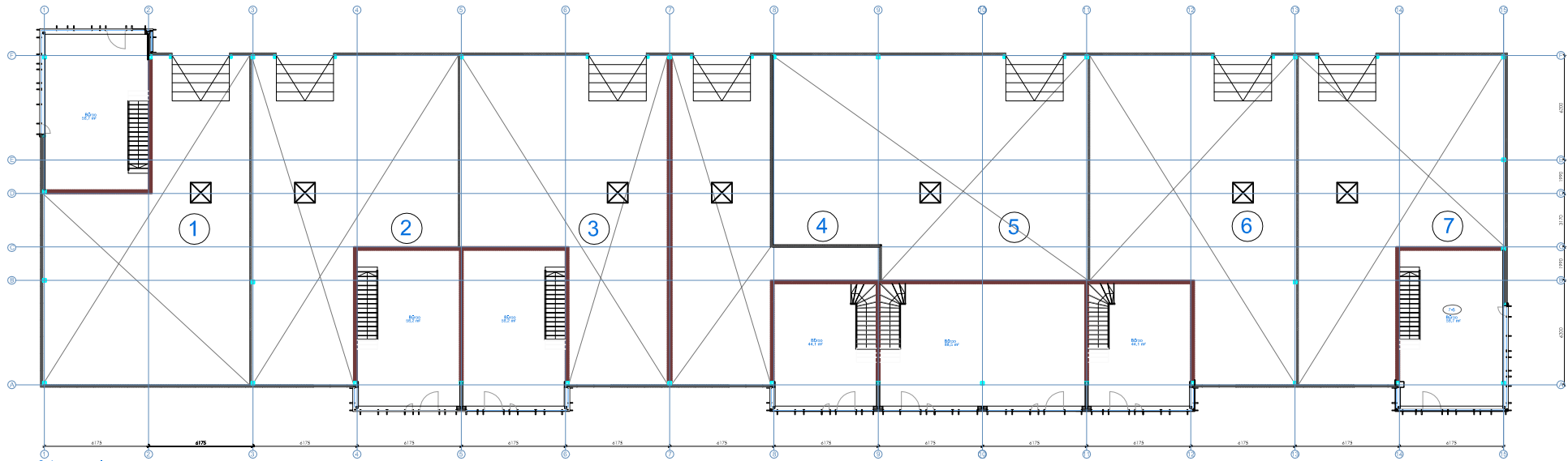
2. korruse plan
